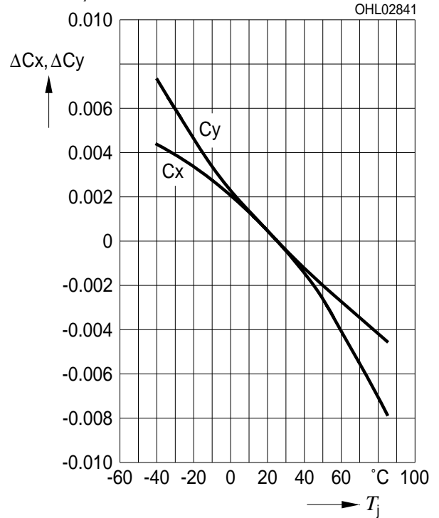
Farbortverschiebung 2) Seite 17 Chromaticity Coordinate Shift 2) page 17 x, y = f(T_j); I_F = 10\text{ mA}
