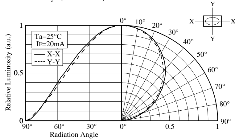
■ Directivity (NSCW335)
