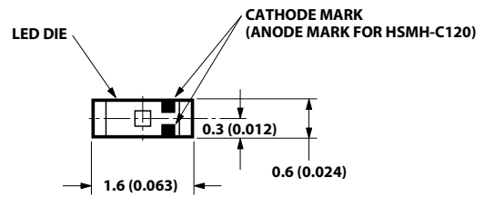
HSMx-C197
